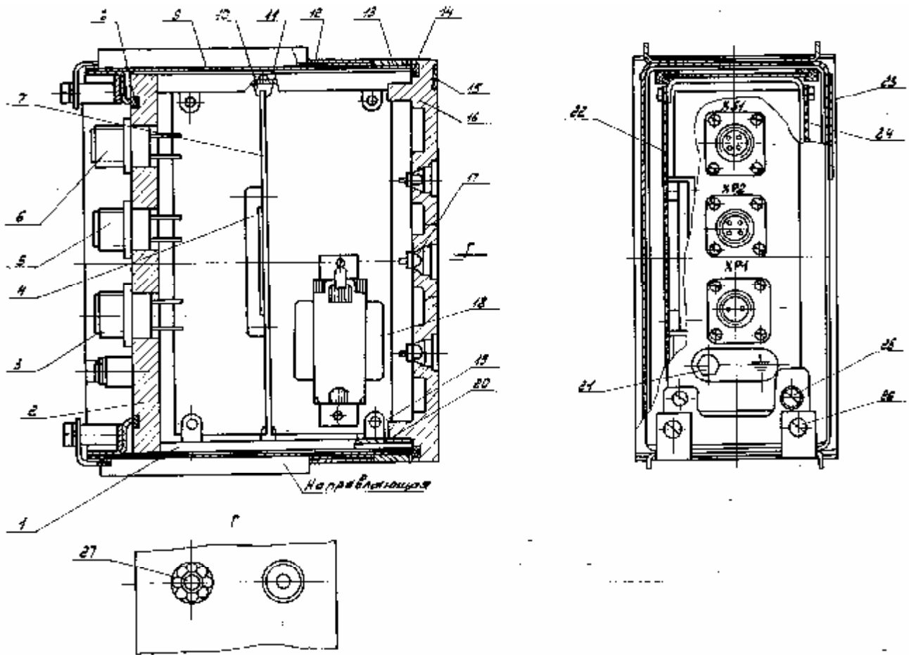
1 – блок электронный; 2- панель задняя; 3, 4, 5, 6 - разъемы; 7 – блок коммутации; 8 - прокладка; 9 – кожух; 10 – обойма; 11, 20 – пластины; 12 – рама; 13 – бандаж; 14 – прокладка; 15, 23 – таблички; 16 – панель передняя; 17 – светодиоды; 18 – трансформатор; 19 – кронштейн; 21 – болт заземления; 22- блок питания; 24 – крышка; 25, 26 – винты; 27 – вставки плавкие.
